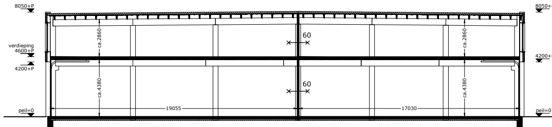
langsdoorsnede
